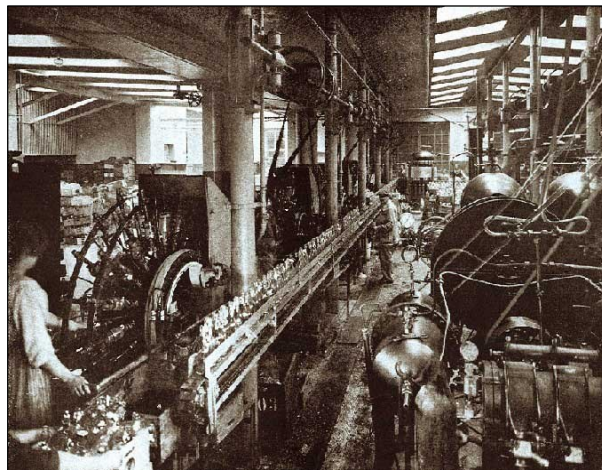
Rotační stroj na mytí lahví v sodovkárně v Karlíně, rok 1927
