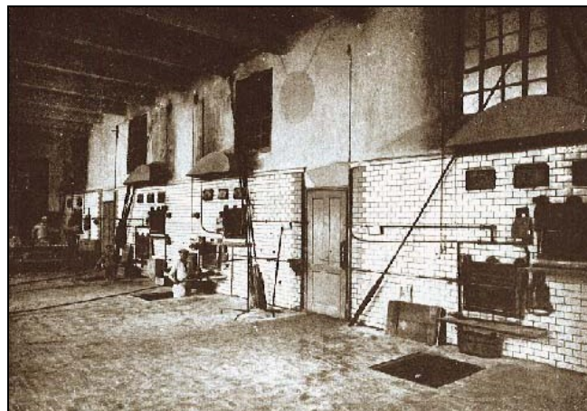
Pekárenská dvorana s parními vyťahovacími pecemi a parní pece pro ruční sázení pečiva, obojí v nové budově pekárny v Holešovicích, 1911
