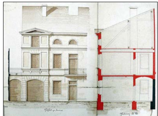
Plán přístavby továrny na hořčici z roku 1885 (SOA)
