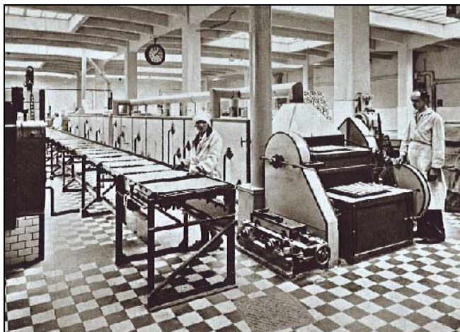
Řetězová pec na topení plynem a stroj na čištění a mazání plechů
